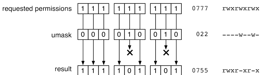
Figure 11.8 umask
