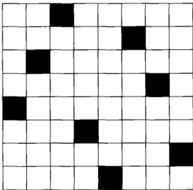
图 4.16 8 \times 8 的国际象棋棋盘上摆着 8 个皇后（黑色小方格），任意两个皇后不在同一行、同一列或者同一对角线上
