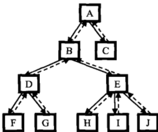
图 7.1 树中的结点有指向父结点的指针，用虚线箭头表示
