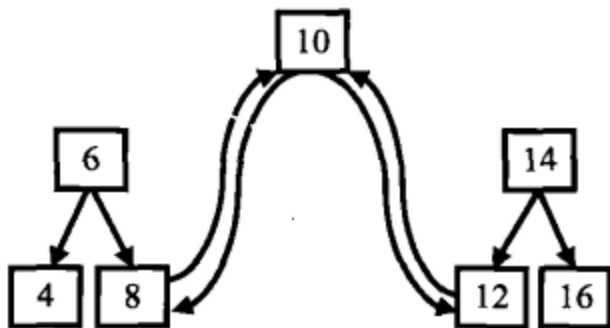
图 4.13 把二叉搜索树看成三部分
